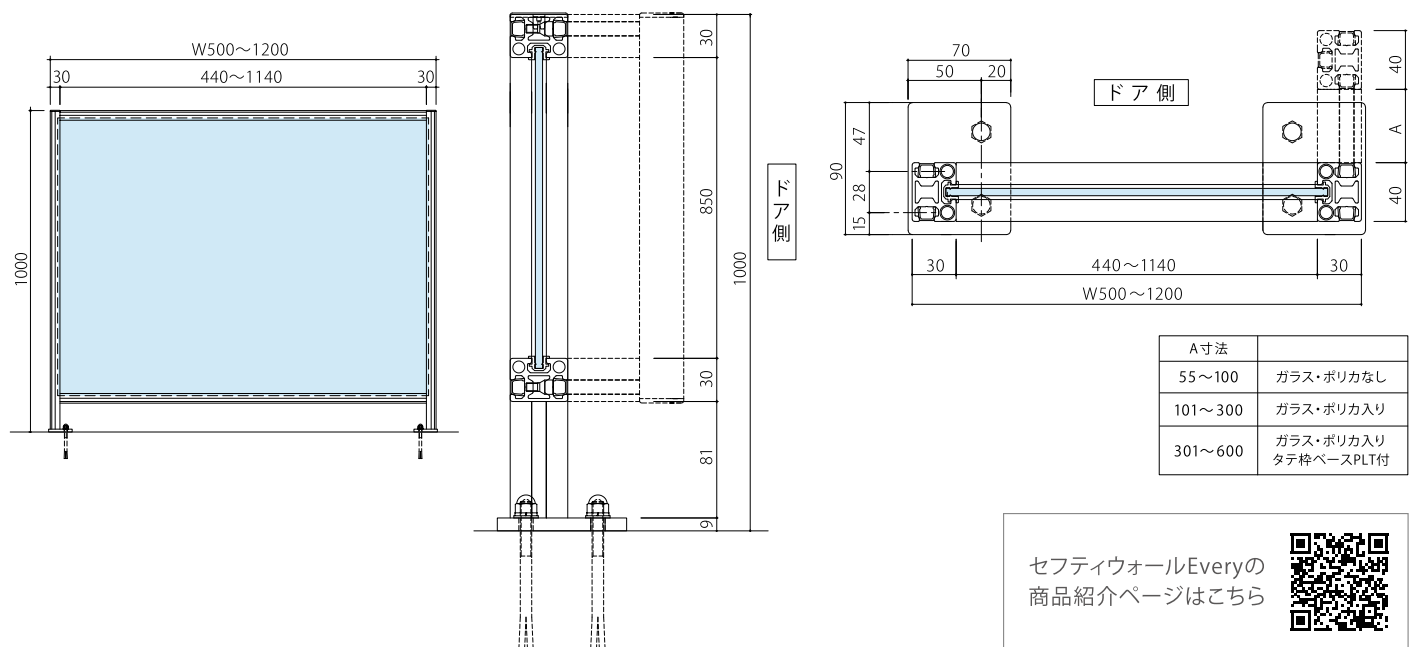
寸法図
