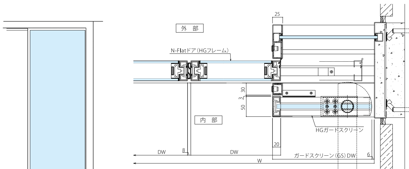
寸法図
