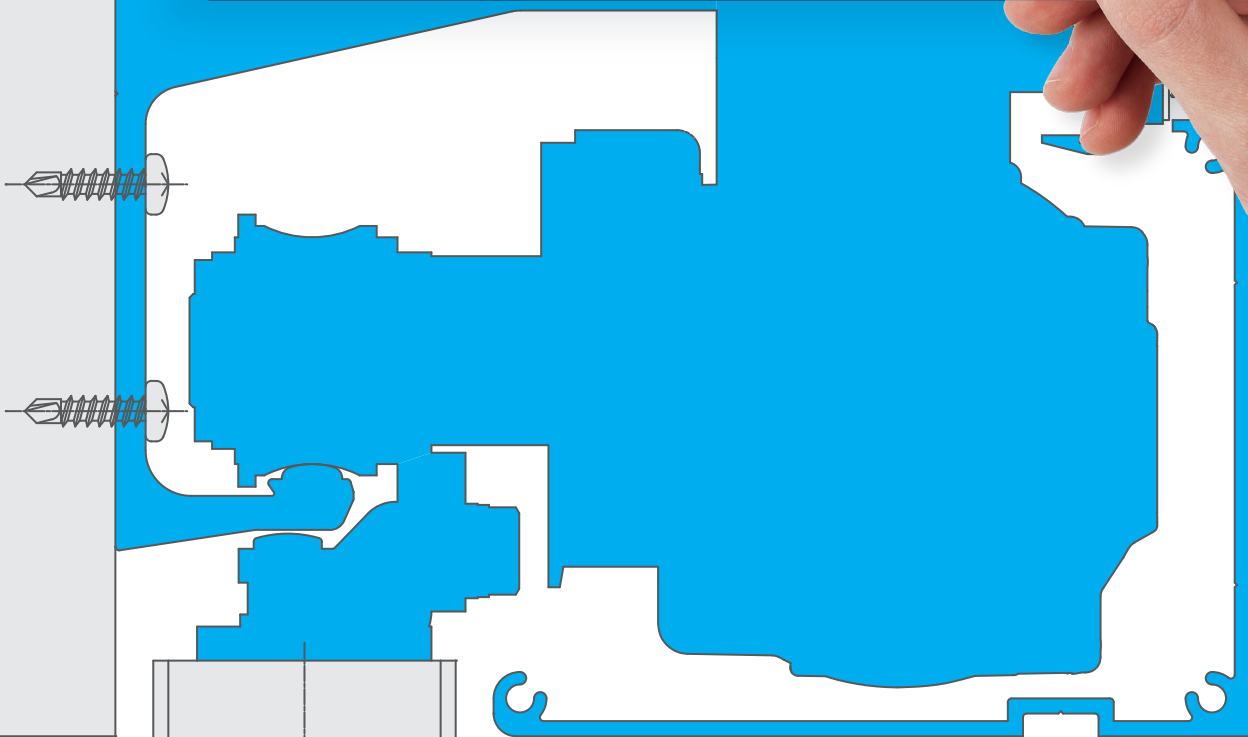
原寸大の断面図
